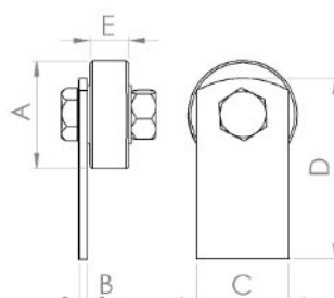
1 rolamento - 1 haste - Inferior
