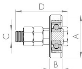
1 rolamento - Porta basculante
