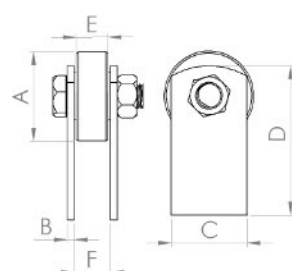
1 rolamento - 2 hastes - Superior
